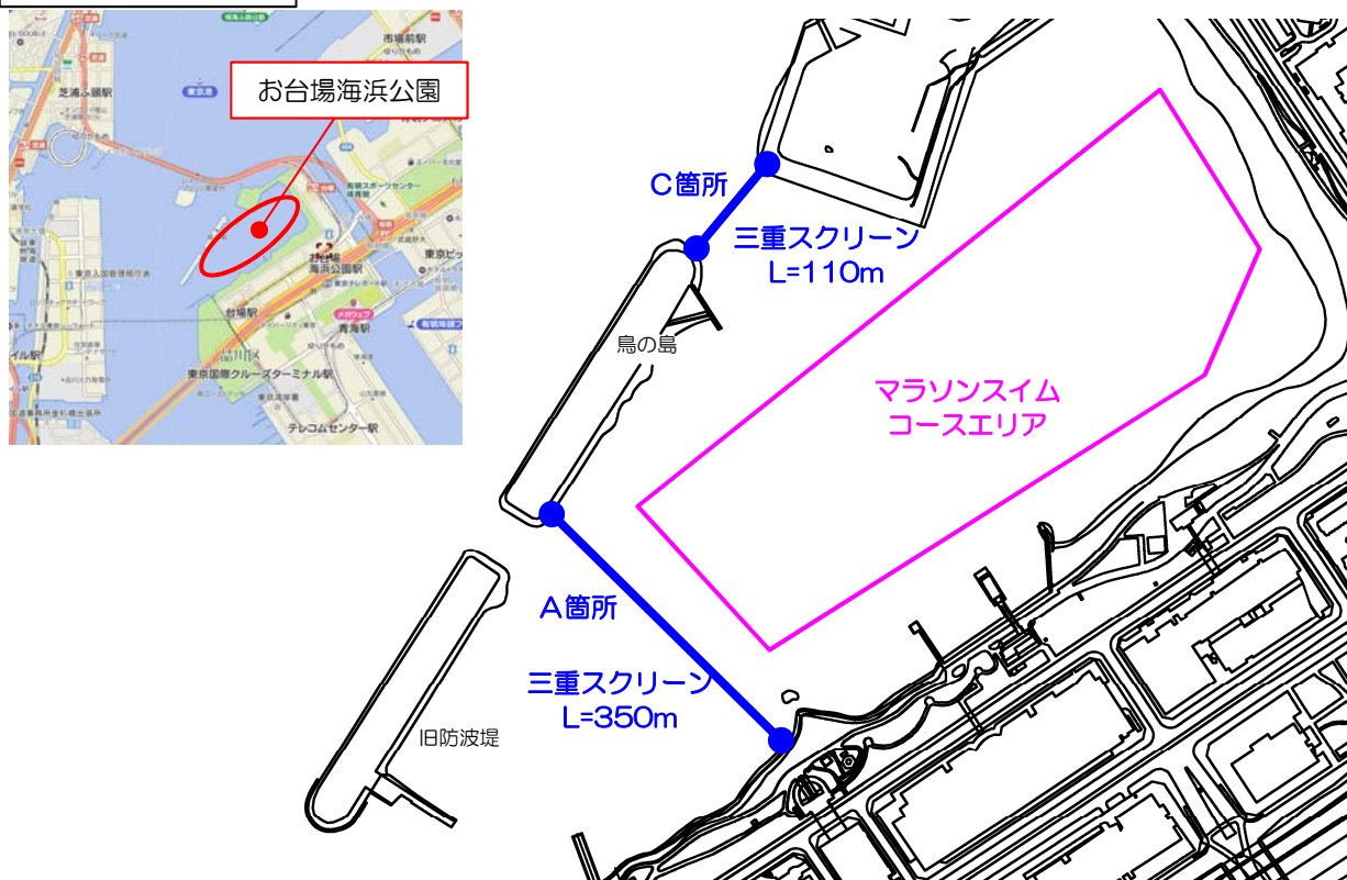
施工位置図
