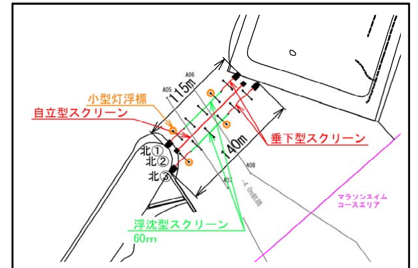
C箇所 スクリーン平面図
