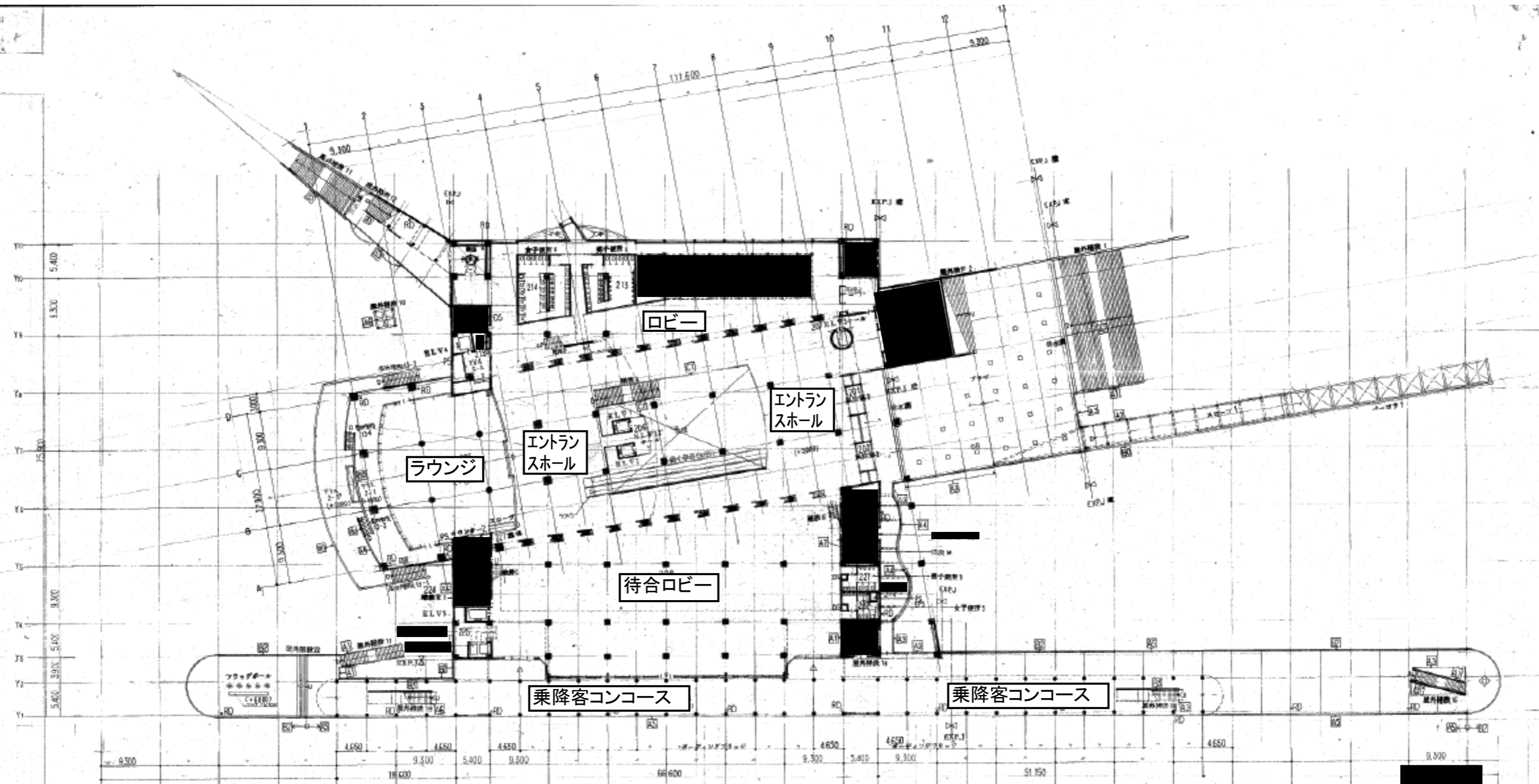
2階平面図
