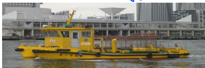
船名 第一清海丸 トン数14トン 平成10年3月竣工 長さ13m 幅6.6m 深さ1.7m 馬力230ps×2基
